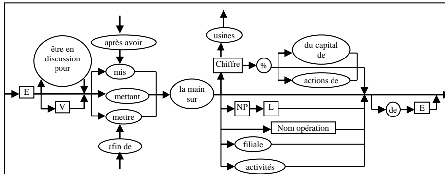
Fig. 4.1 : exemple d'automate d'extraction d'information [AMA 01]
