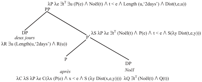
Figure 2. Compositional calculus of the semantics of deux jours après Noël
