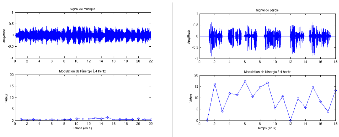
FIG. 3.4 – Modulation de l'énergie à 4 Hertz pour la musique (extrait de Mozart) et la parole (6 phrases de parole lue).
