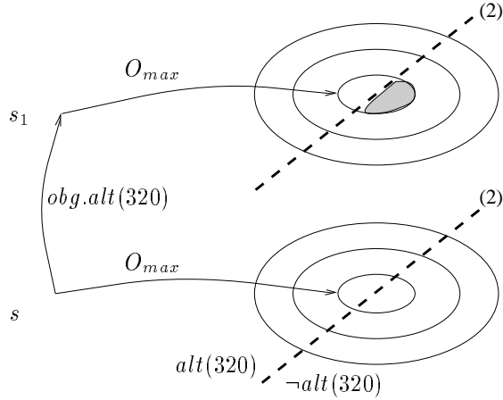
Figure 3: Evolution des obligations après obg.alt(320) . Cas où alt(320) n'était pas obligatoire.
